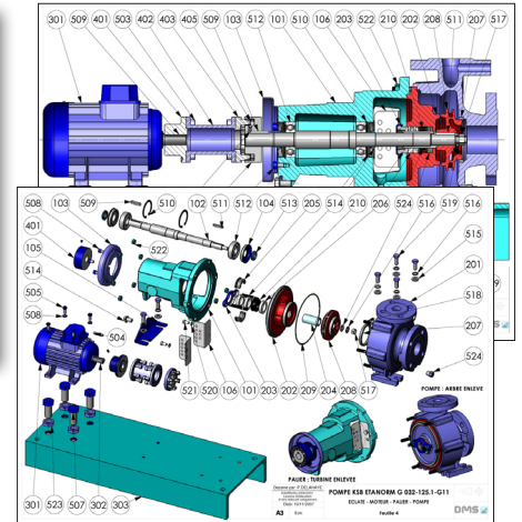
Modélisation 3D sous Solidworks
